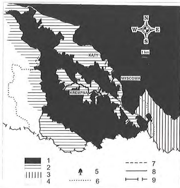
Ryc. 3. Obszary chronione w dorzeczu górnej Wisłoki.
