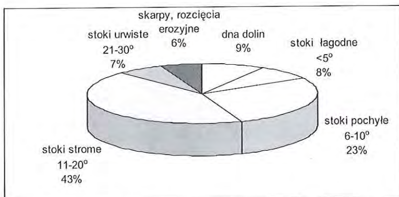
Ryc. 2. Formy rzeźby terenu w otoczeniu planowanego zbiornika Kąty-Myscowa na Wisłocy (w granicach zlewni bezpośredniej). Źródło: Sroczyński, Józefko 2002.
